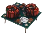
FLT007A0Z 25.4 x 25.4 x 12.2 mm
