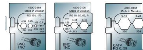
Art.nr. 4300-3140 RG 174, 179 BNC, TNC Art.nr. 4300-3136 RG 58, 59, 62, 71 BNC, TNC kontakti Art.nr. 4300-3138 RG 6, 59 CATV kontakti
