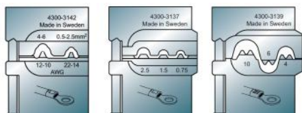
Art.nr. 4300-3142 0.5 - 6 mm 2 Art.nr. 4300-3137 0.5 - 2.5 mm 2 Art.nr. 4300-3139 4 - 10 mm 2
