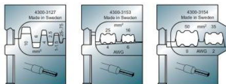
Art.nr. 4300-3127 0.25-10 mm 2 Art.nr. 4300-3153 16 - 25 mm 2 Art.nr. 4300-3154 35 - 50 mm 2
