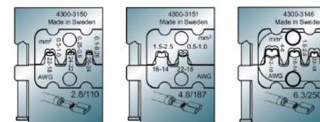
Art.nr. 4300-3150 0.1 - 1 mm 2 2.8/110 kontakti Art.nr. 4300-3151 0.5 - 2.5 mm 2 4.8/187 kontakti Art.nr. 4300-3146 0.5 - 6 mm 2 6.3/250 kontakti
