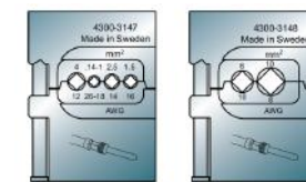
Art.nr. 4300-3147 0.14 - 4 mm 2 Art.nr. 4300-3148 6 - 10 mm 2
