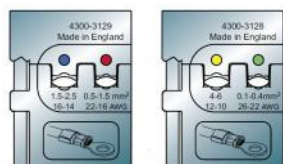
Art.nr. 4300-3129 0.5 - 2.5 mm 2 Art.nr. 4300-3128 0.1-0.4, 4-6 mm 2
